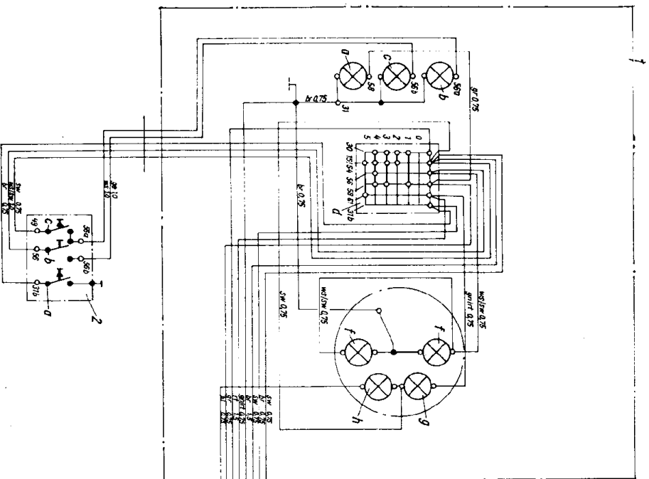
Bild 80. Schaltplan ohne Blinkleuchten (TS 125 und 150)
