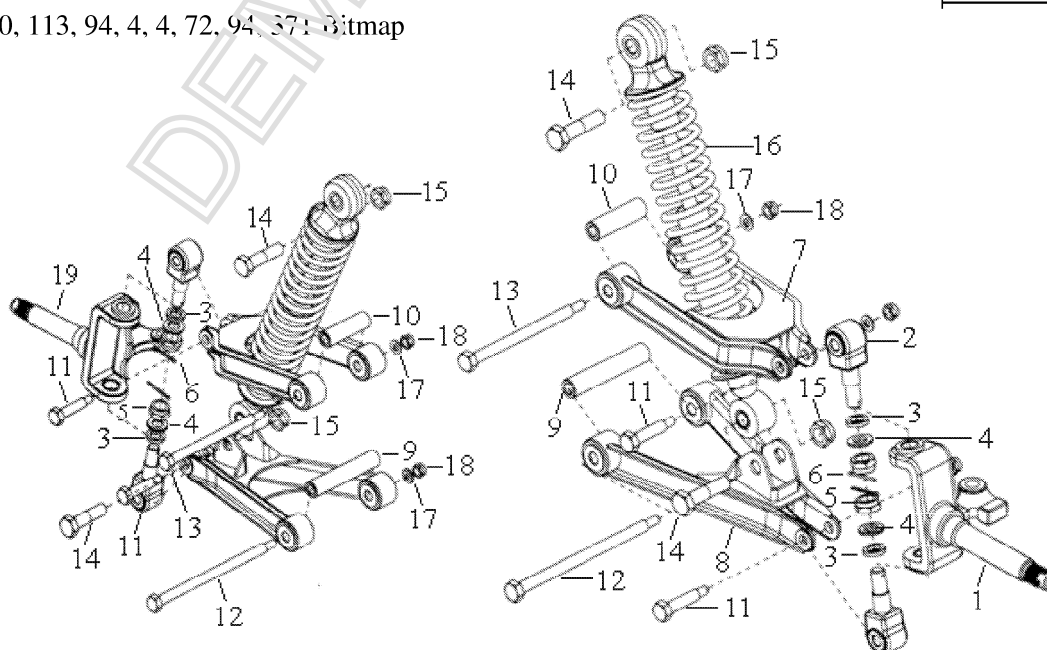
FIG.10 DUAL A-ARM
