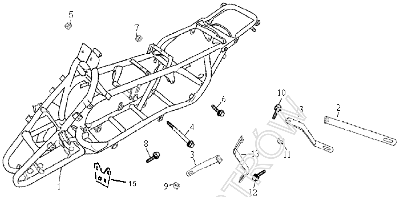
FIG.10 FRAME
